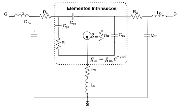
Figura 2. Circuito eléctrico equivalente del transistor GaN utilizado
