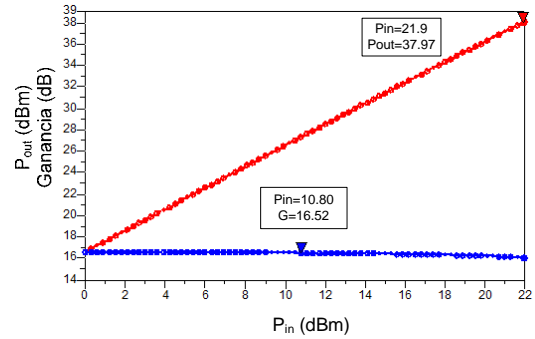
Figura 10. Respuesta P_{in} Vs P_{out} del AP clase B diseñado
