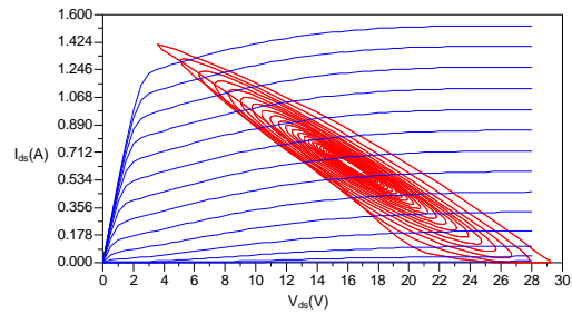
Figura 5. Recta de carga estimada del AP Clase A diseñado.
