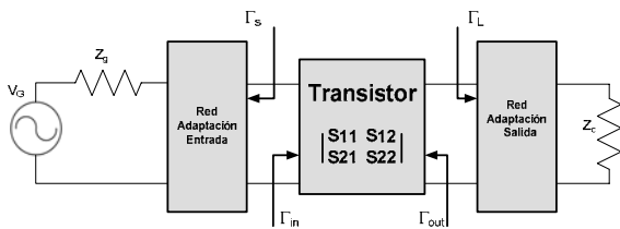
Figura 4. Esquema de un Amplificador.
