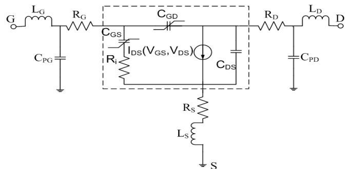
Figura 3. Circuito Eléctrico Equivalente del transistor GaN utilizado.
