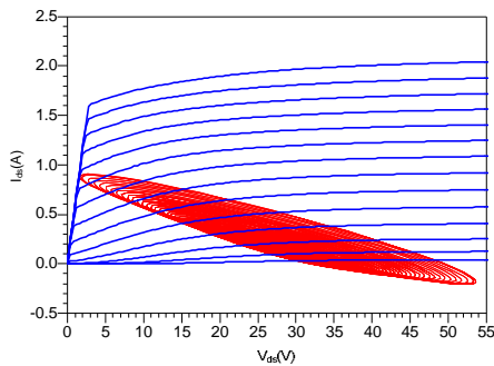
Figura 8. Recta de carga estimada del AP Clase B diseñado.
