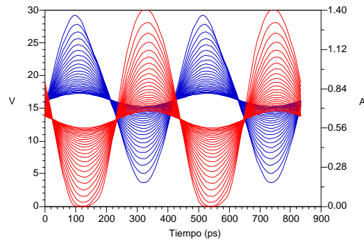
Figura 6. Formas de ondas presentadas en la salida del AP clase A.
