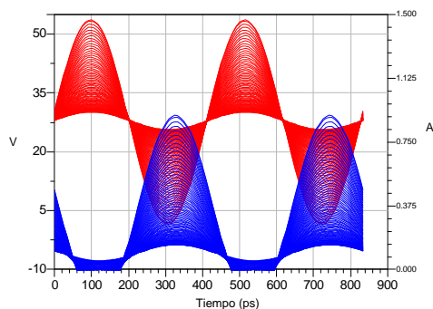
Figura 9. Formas de onda presentadas en la salida del AP clase B diseñado.
