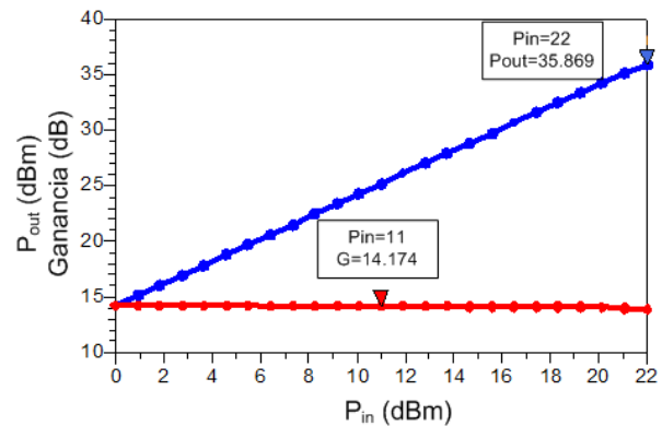
Figura 7. Respuesta P_{in} Vs P_{out} del AP clase A diseñado
