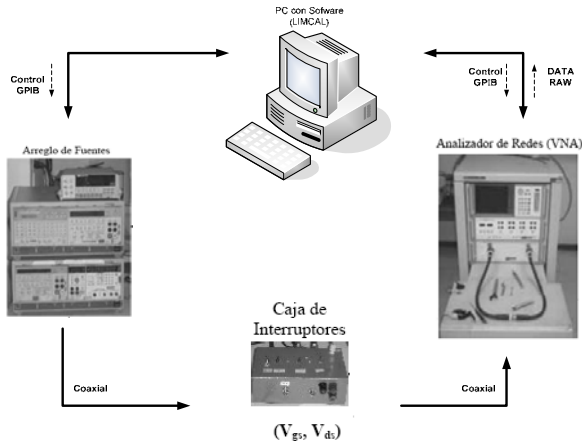
Figura 1. Banco de medición para la caracterización de Transistores GaN
